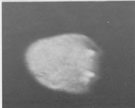
Jupiter-Mond Europa: von Eis umschlossen Jupiter-Mond Amalthea: kleinster der 5 Großen
