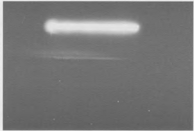
23.6.1979, 04.25 h: Eines der Energieschiffe etwa 2 km vom Center entfernt vor dem nordwestlichen Horizont.
